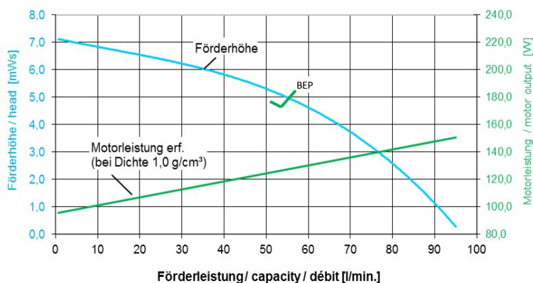
Kennlinien RT-VC100 - Typ 7/80
